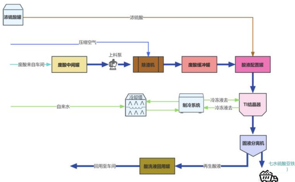
图 7 酸洗车间硫酸循环利用系统设施图
