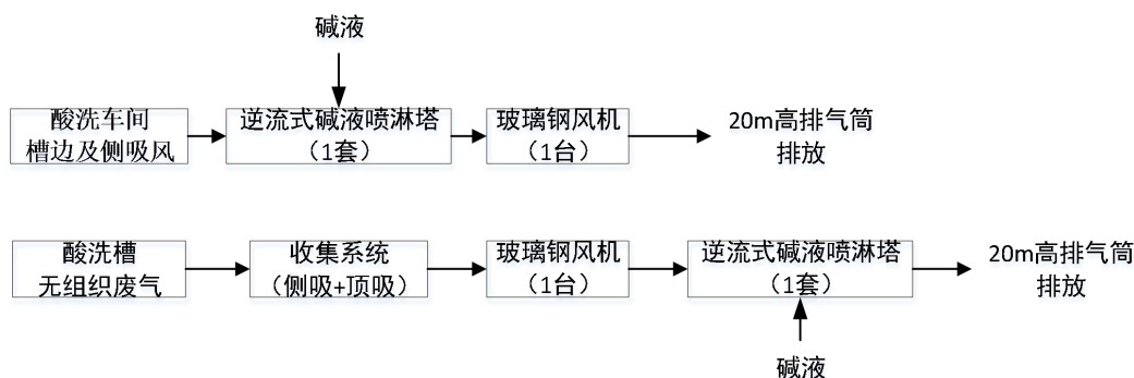
图 6 酸洗车间废气处理设施图
